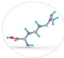
Peptide
